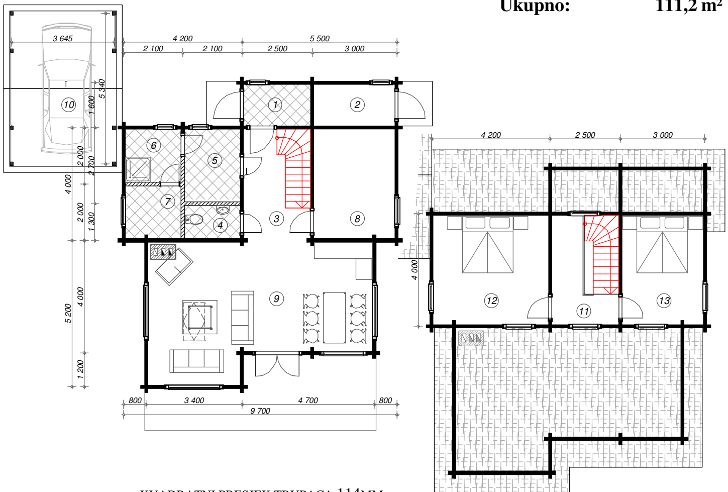
KVADRATNI PRESJEK TRUPACA 114MM
